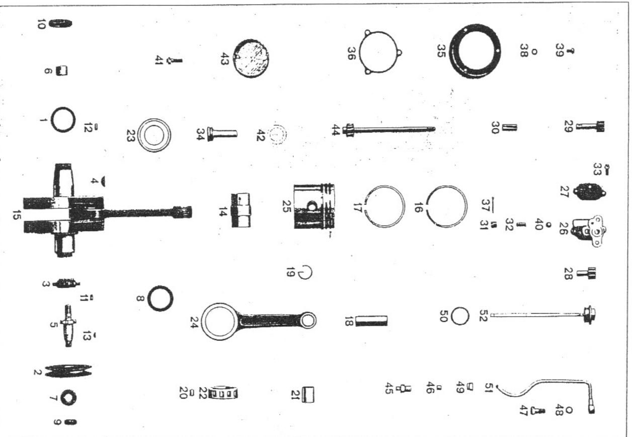
Tafel 12 Kurbelwelle, Kolben und Pleuel, Ölpumpe, Öldruckschmierung, Ölkontrolle
